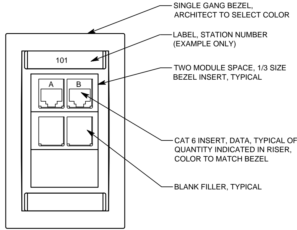
5 TYP VOICE-DATA OUTLET NO SCALE
