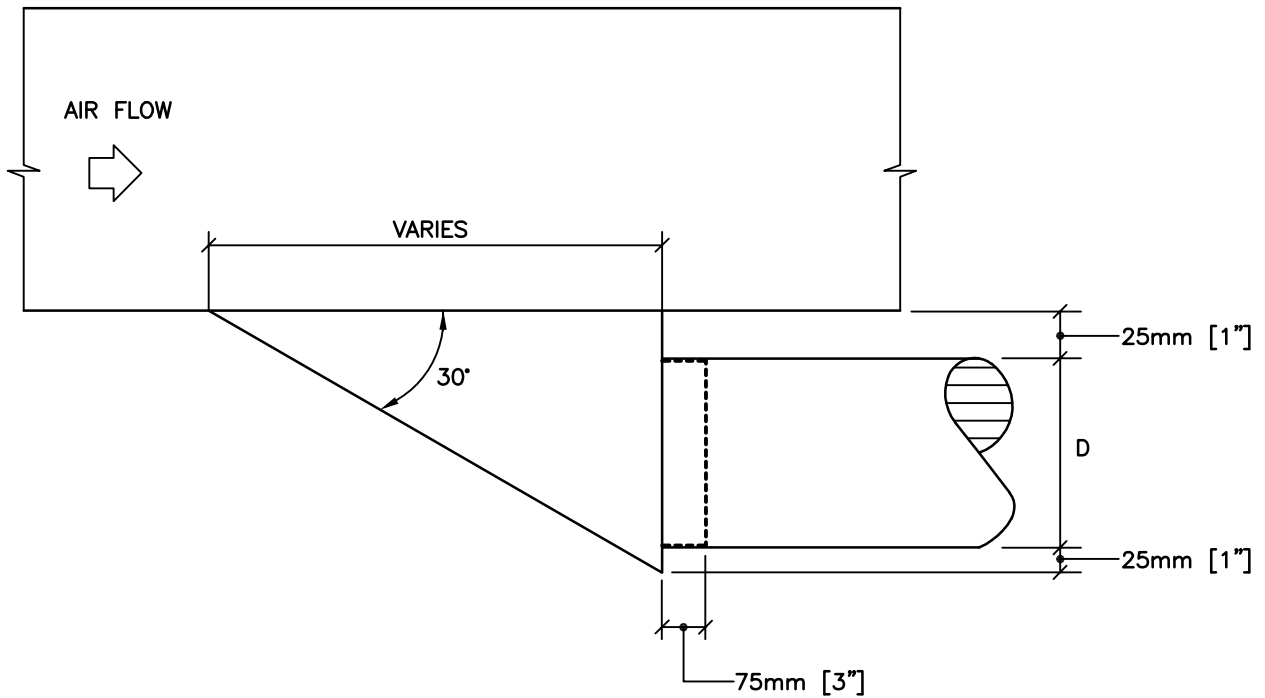
ELEVATION
